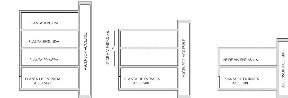
Figura 1. Ejemplos de exigibilidad de ascensor accesible o rampa accesible en edificios de vivienda.
