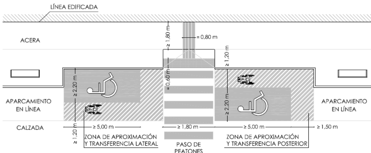
Figura 5. Posible configuración de plazas en línea
